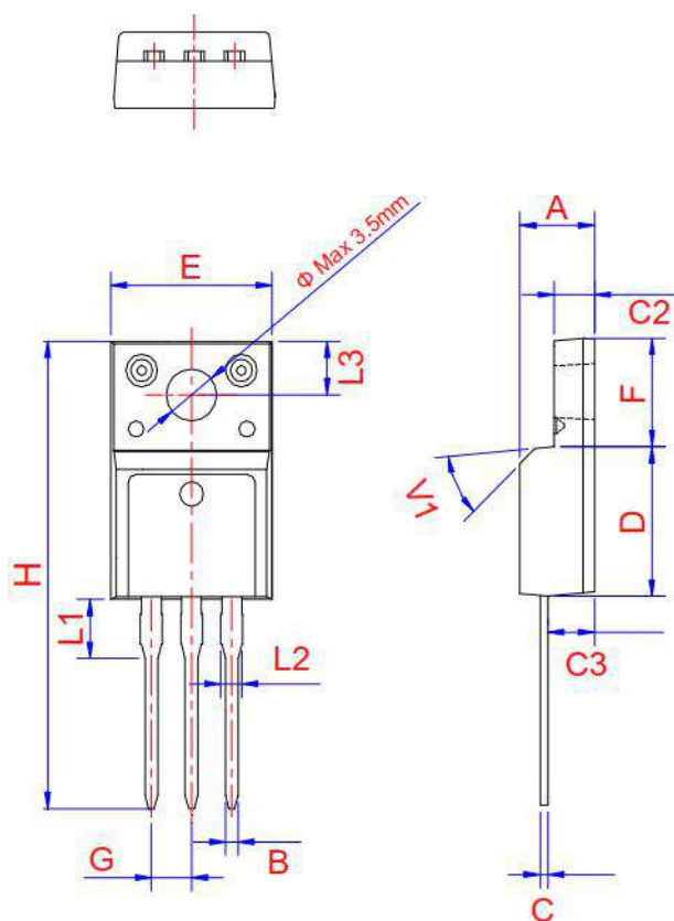
TO-220F Ins
