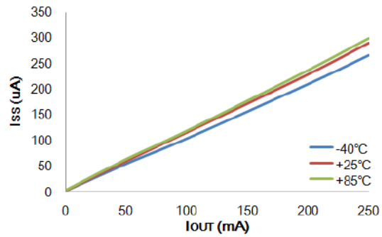
I_{SS} vs I_{OUT} : HT73L10 ( V_{IN}=2.3V )
