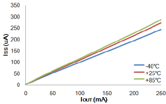
I_{SS} vs I_{OUT} : HT73L09 ( V_{IN}=2.3V )
