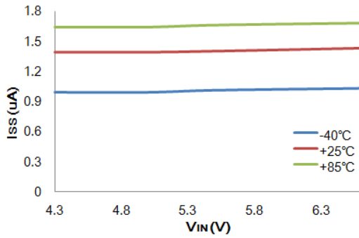
I_{SS} vs V_{IN} : HT73L33 ( I_{OUT}=0mA )
