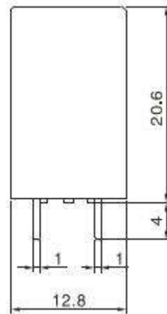
线路图 (底视图) Wiring Diagram (Bottom View)
