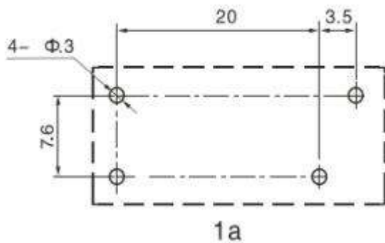
安装孔位图(底视图)
