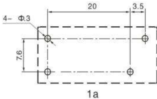
安装孔位图(底视图)
