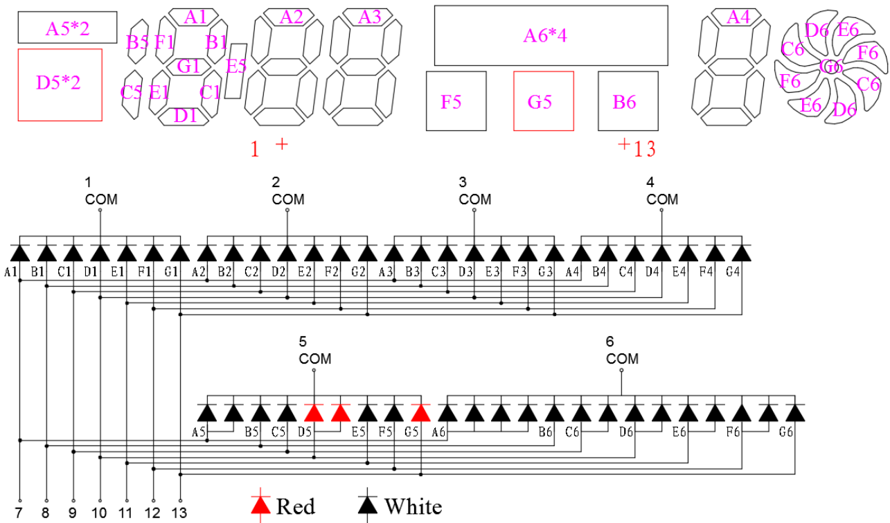
线路图 (circuit)
