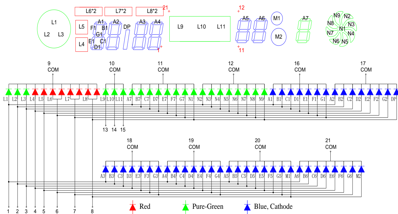
线路图 (circuit)
