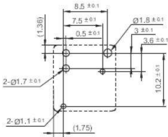
PCB 安装图
