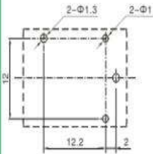
安装孔位图(底视图)
