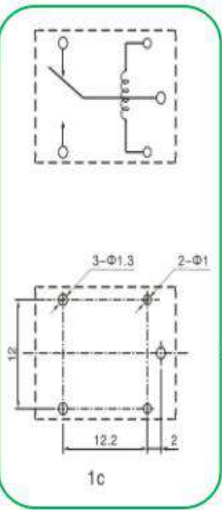
接线图(底视图)
