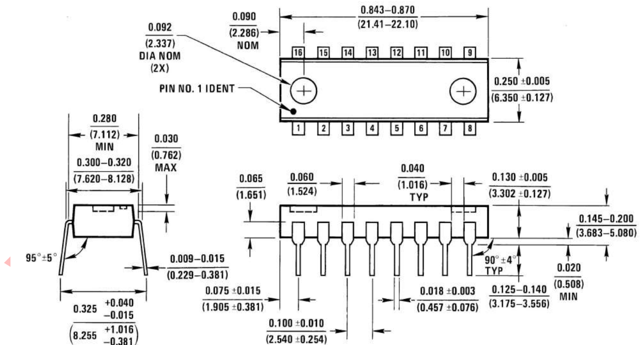
图 DIP16 封装尺寸图
