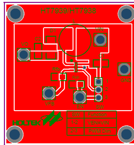
Top Layer
