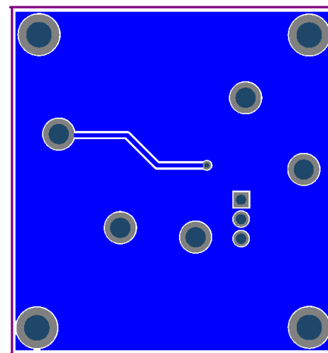
Bottom Layer
