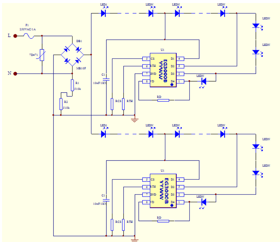
图 3. EG3000B 并联使用方案
