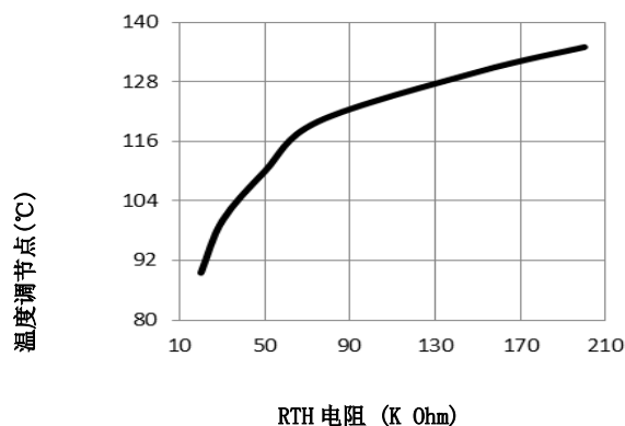
IC 过温保护点与 RTH 电阻关系曲线
