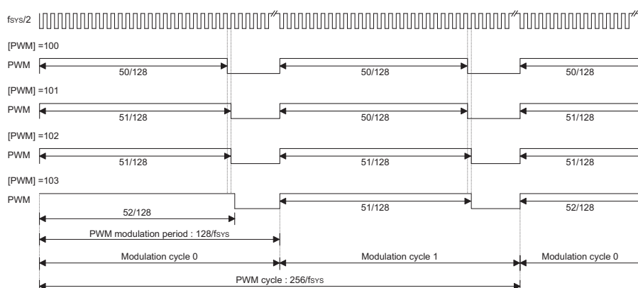
7+1 PWM Mode
