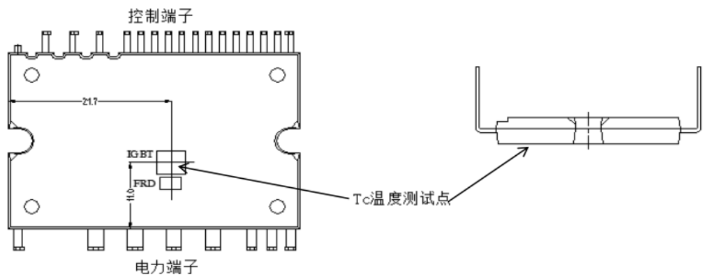
图 4：壳温 T_c 测试点 Fig 4: Case Temperature Measurement
