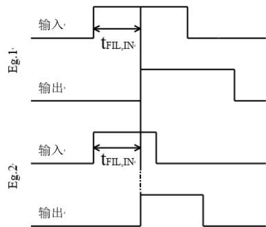
图 9：增强型输入滤波 9: Enhanced input filtering
