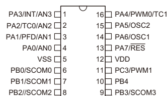
HT46R066 16 DIP-A/NSOP-A
